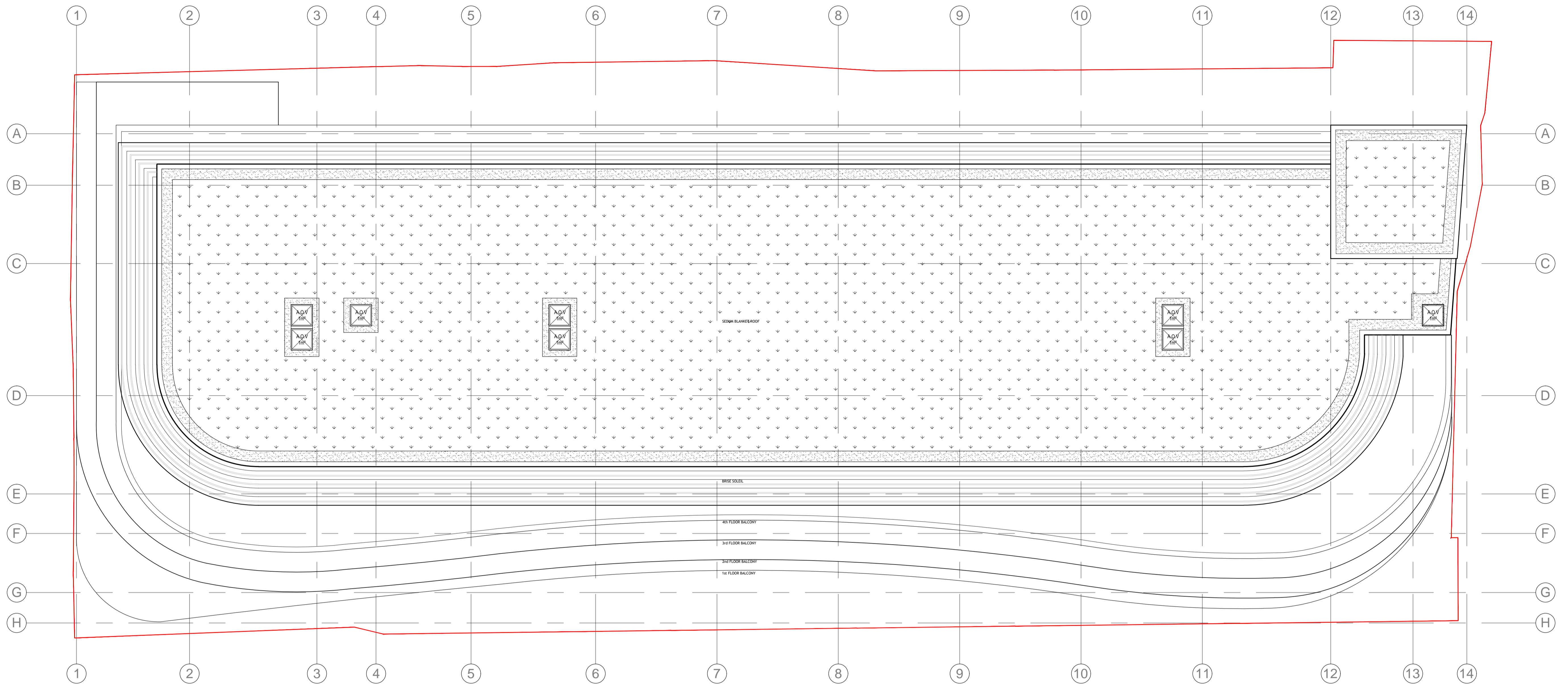
R O O F P L A N S c a l e 1 : 1 0 0
